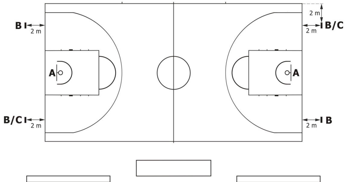
Bild 3.1 Anordnung der Wurfuhr-Anzeigeräte
